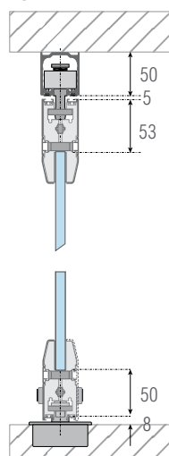
Corte B PUERTA ABATIBLE
