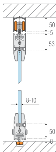
Corte A PUERTA PLEGABLE
