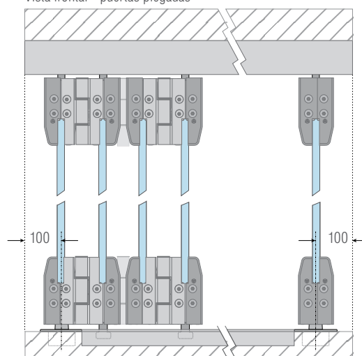
Vista frontal - puertas plegadas
