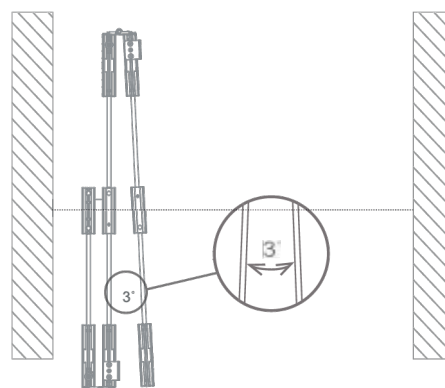
Vista Superior - Puertas Plegadas
